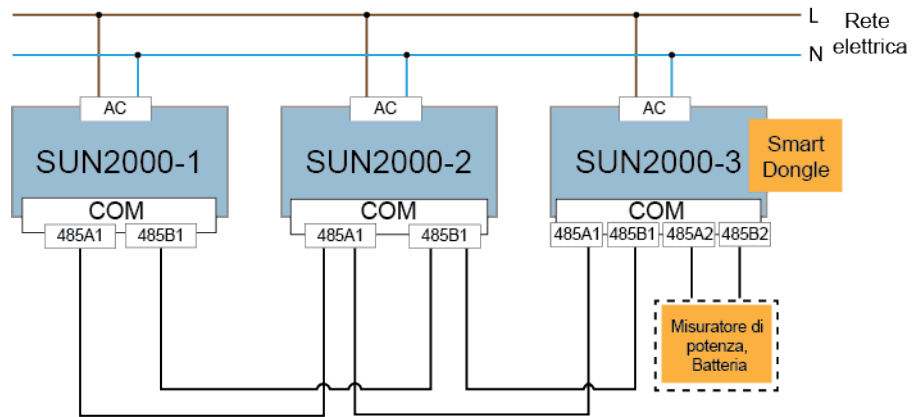
Figura 5-21 Collegamento rete in fase
