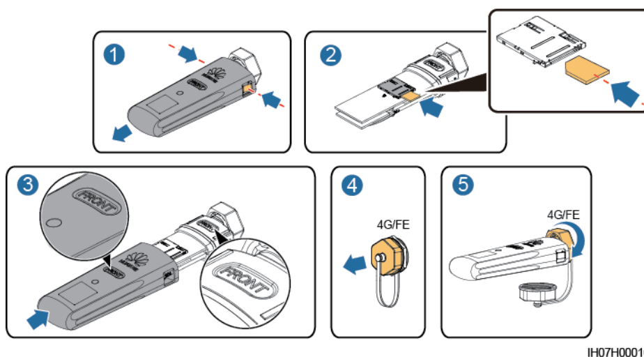
Figura 5-5 Installazione di uno Smart Dongle 4G
