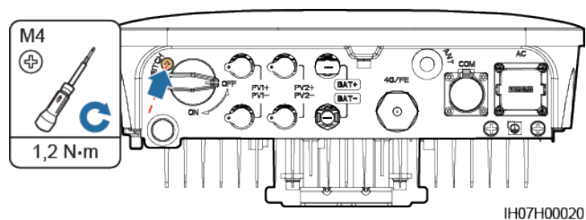
Figura 4-15 Installazione di una vite di bloccaggio per l'interruttore CC
