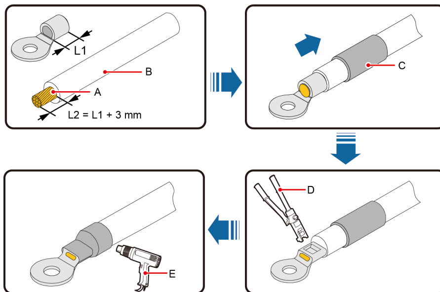
Figura 5-2 Crimpatura di un terminale OT
