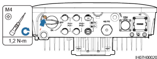
Figura 4-10 Installazione di una vite di bloccaggio per l'interruttore CC
