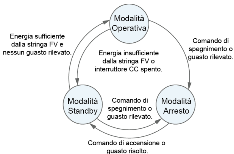
Figura 2-8 Modalità di funzionamento
