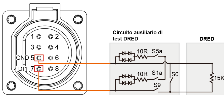
Figura 7-19 Schema di cablaggio per funzione DRM
