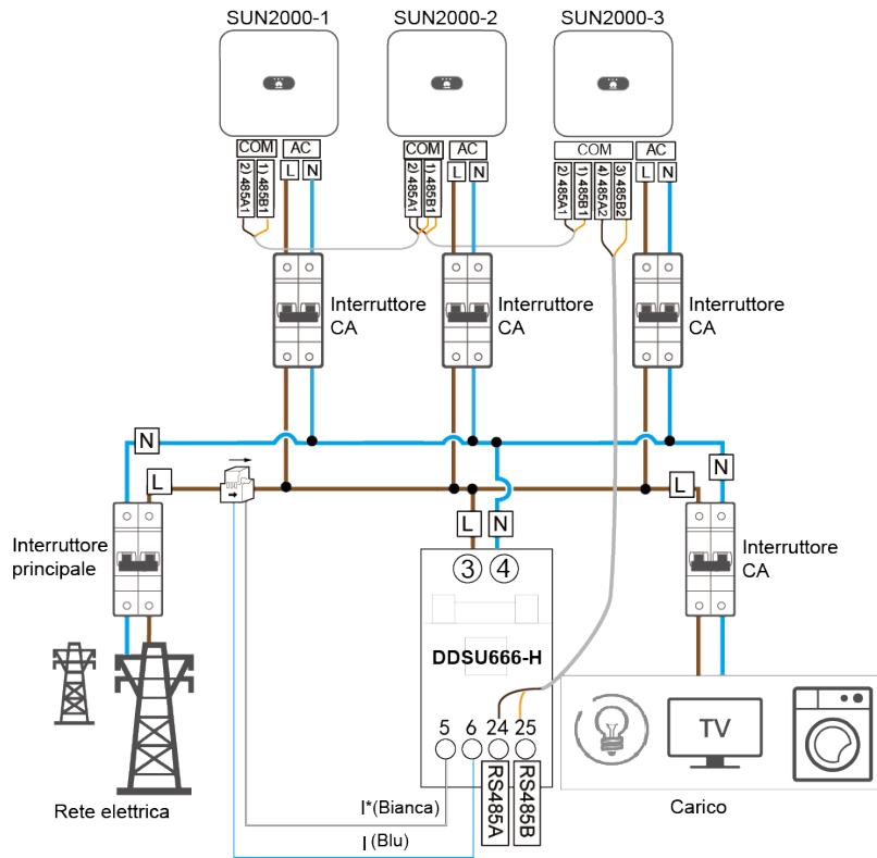
Figura 5-22 Collegamento dei cavi allo Smart Power Sensor (collegamento rete in fase)
