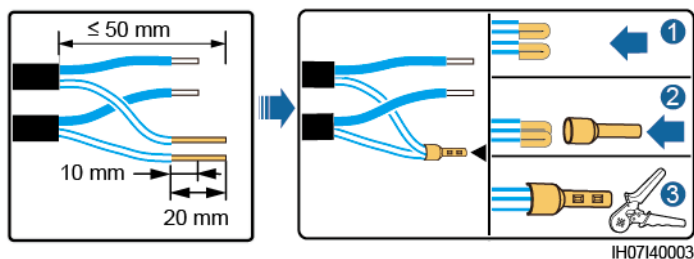
Figura 5-25 Crimpatura di due cavi di segnale
