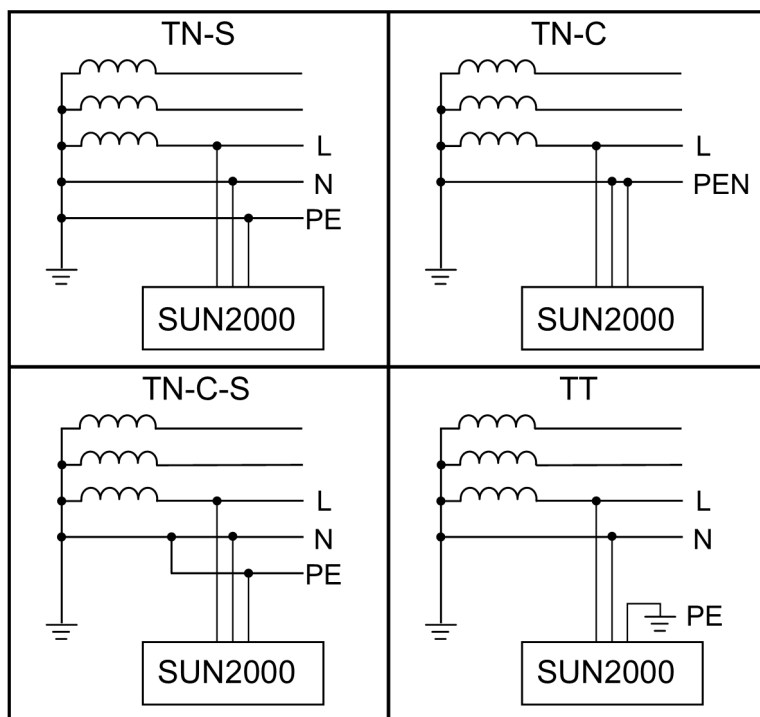
Figura 2-4 Tipi di rete elettrica
