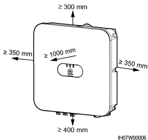
Figura 4-2 Spazio di installazione
