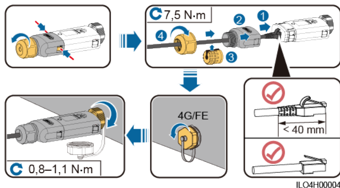
Figura 5-6 Installazione di uno Smart Dongle WLAN-FE (per comunicazioni FE)
