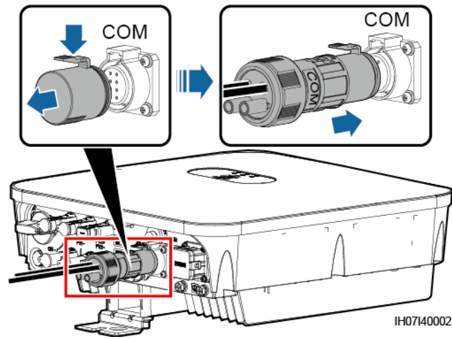
Figura 5-29 Fissaggio di un connettore di segnale
