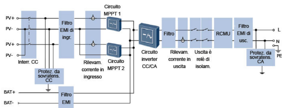
Figura 2-7 Diagramma schematico
