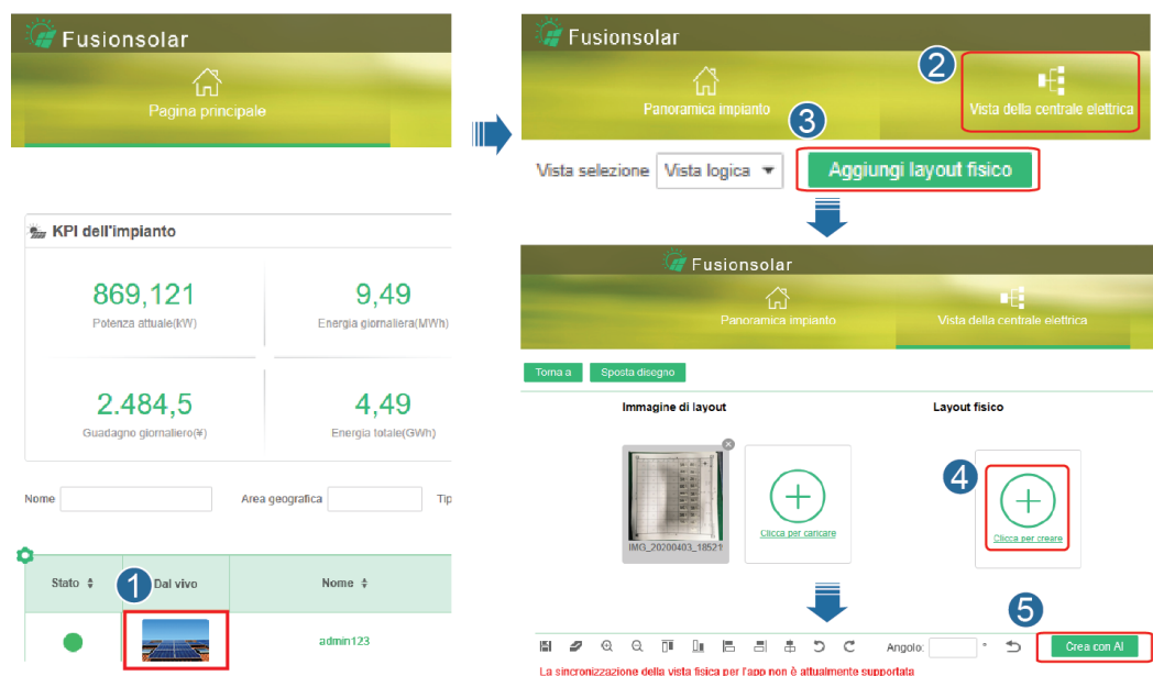
Figura 7-7 Progettazione layout fisico dei moduli FV
