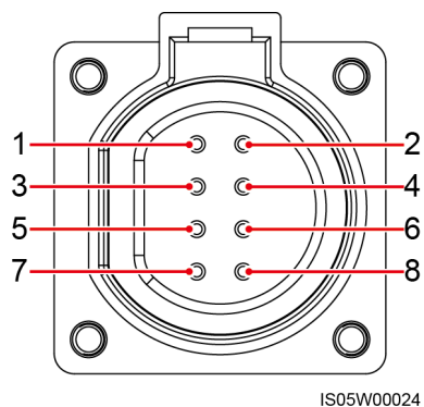
Figura 5-18 Porte dei cavi di segnale
