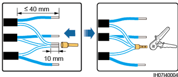
Figura 5-26 Crimpatura di tre cavi di segnale
