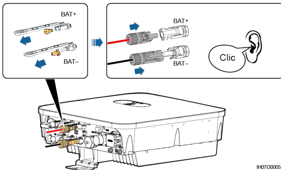
Figura 5-17 Collegamento dei cavi della batteria
