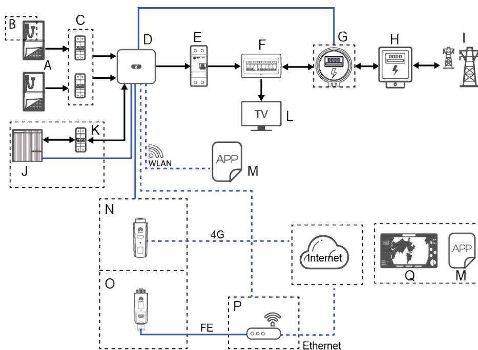
Figura 2-2 Scenario SUN2000 singolo (i riquadri tratteggiati indicano le configurazioni facoltative)
