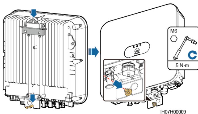
Figura 4-11 Serraggio dei dadi
