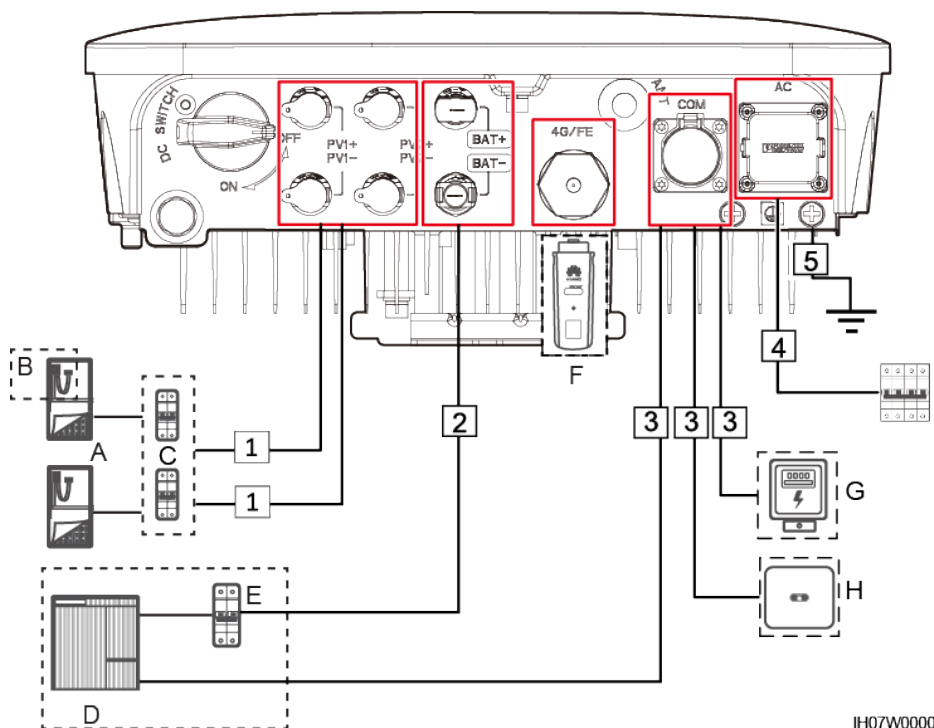
Figura 5-1 Collegamenti dei cavi del SUN2000 (i riquadri tratteggiati indicano le configurazioni facoltative)
