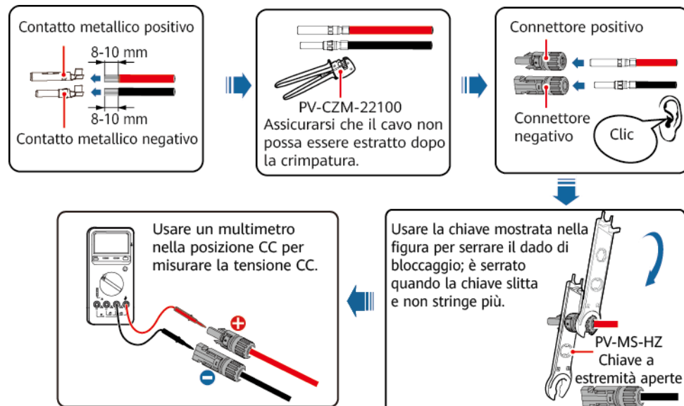
Figura 5-14 Assemblaggio di un connettore CC
