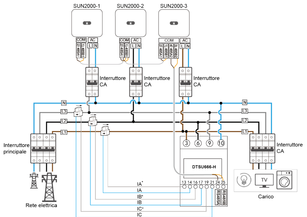
Figura 5-24 Collegamento dei cavi allo Smart Power Sensor (collegamento rete trifase bilanciato)
