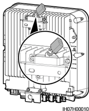
Figura 4-12 Installazione di un lucchetto antifurto
