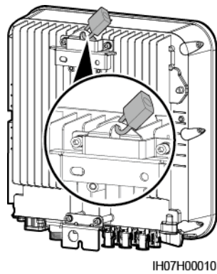
Figura 4-17 Installazione di un lucchetto antifurto
