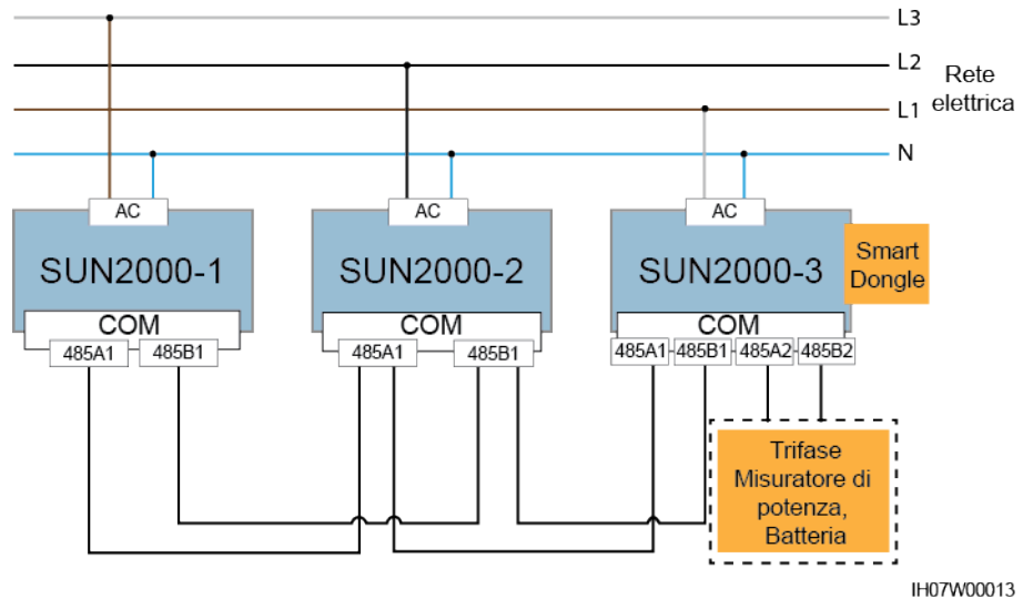
Figura 5-23 Collegamento rete trifase bilanciato
