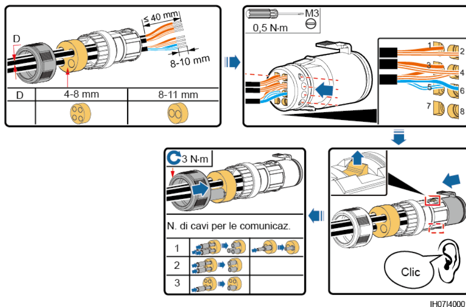
Figura 5-28 Assemblaggio di un connettore di segnale (SUN2000 in cascata)
