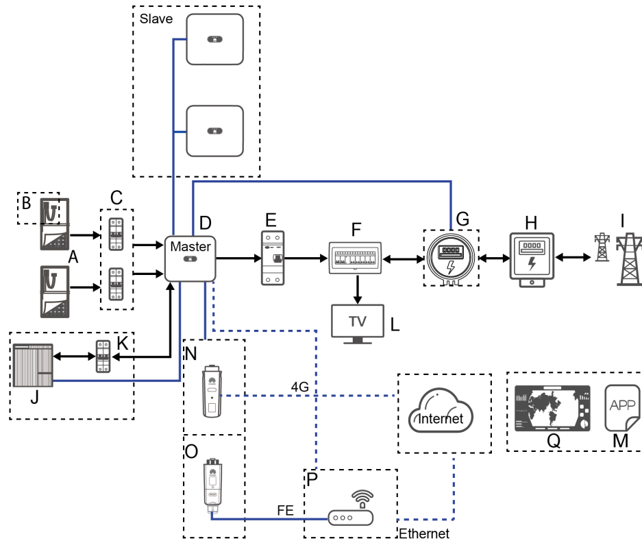
Figura 2-3 Scenario SUN2000 in cascata (i riquadri tratteggiati indicano le configurazioni facoltative)
