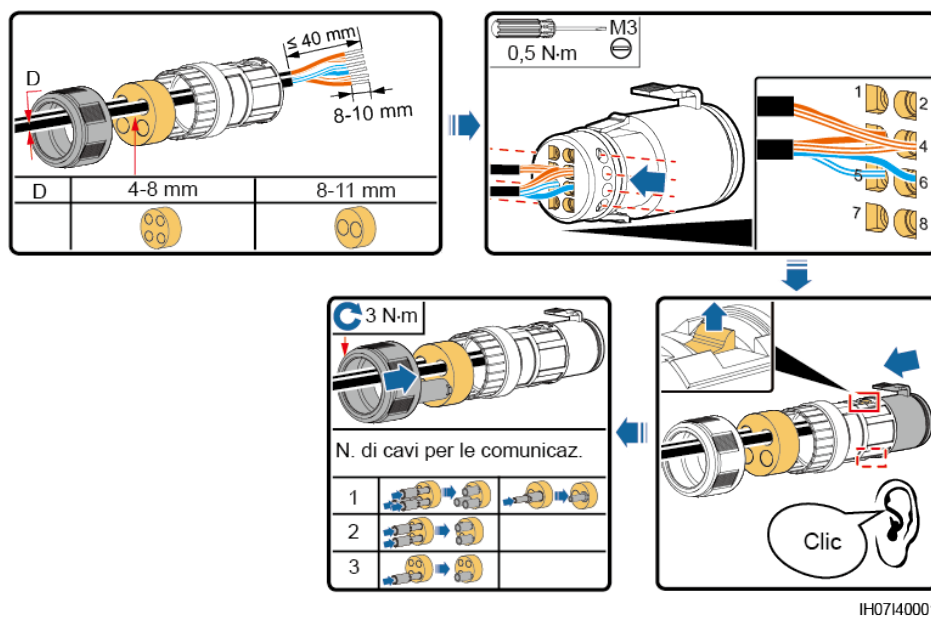
Figura 5-27 Assemblaggio di un connettore di segnale (SUN2000 singolo)
