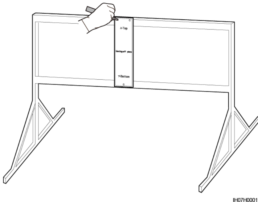
Figura 4-13 Determinazione della posizione dei fori
