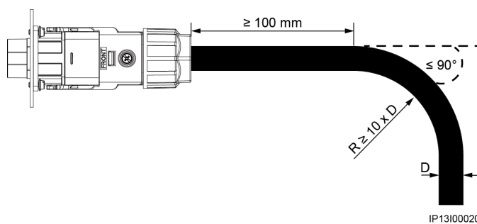
Figura 5-11 Requisiti di cablaggio
