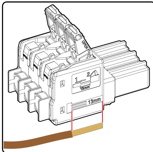
Figura 5-9 Lunghezza per la spelatura del cavo
