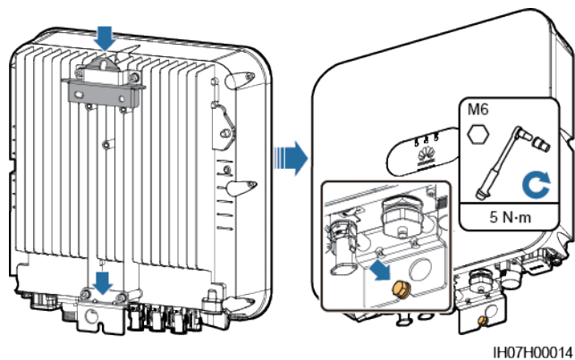
Figura 4-16 Serraggio dei gruppi di bulloni
