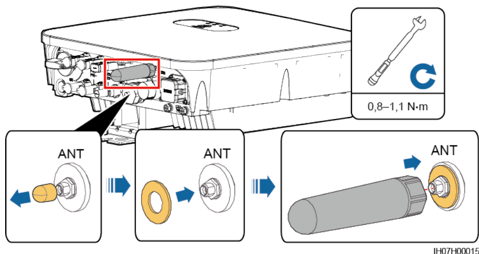
Figura 5-4 Installazione di un'antenna WLAN
