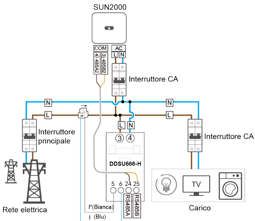
Figura 5-20 Collegamento dei cavi allo Smart Power Sensor (SUN2000 singolo)
